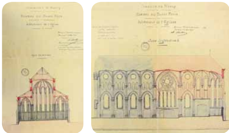
Les plans de l'église Saint-Roch établis par l'architecte Maillard de 1872 à 1875.
